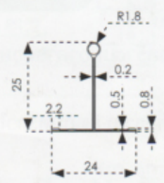
โครงคร่าวหลัก MAIN RUNNER (สิทธิบัตรการออกแบบเลขที่ 17357)
